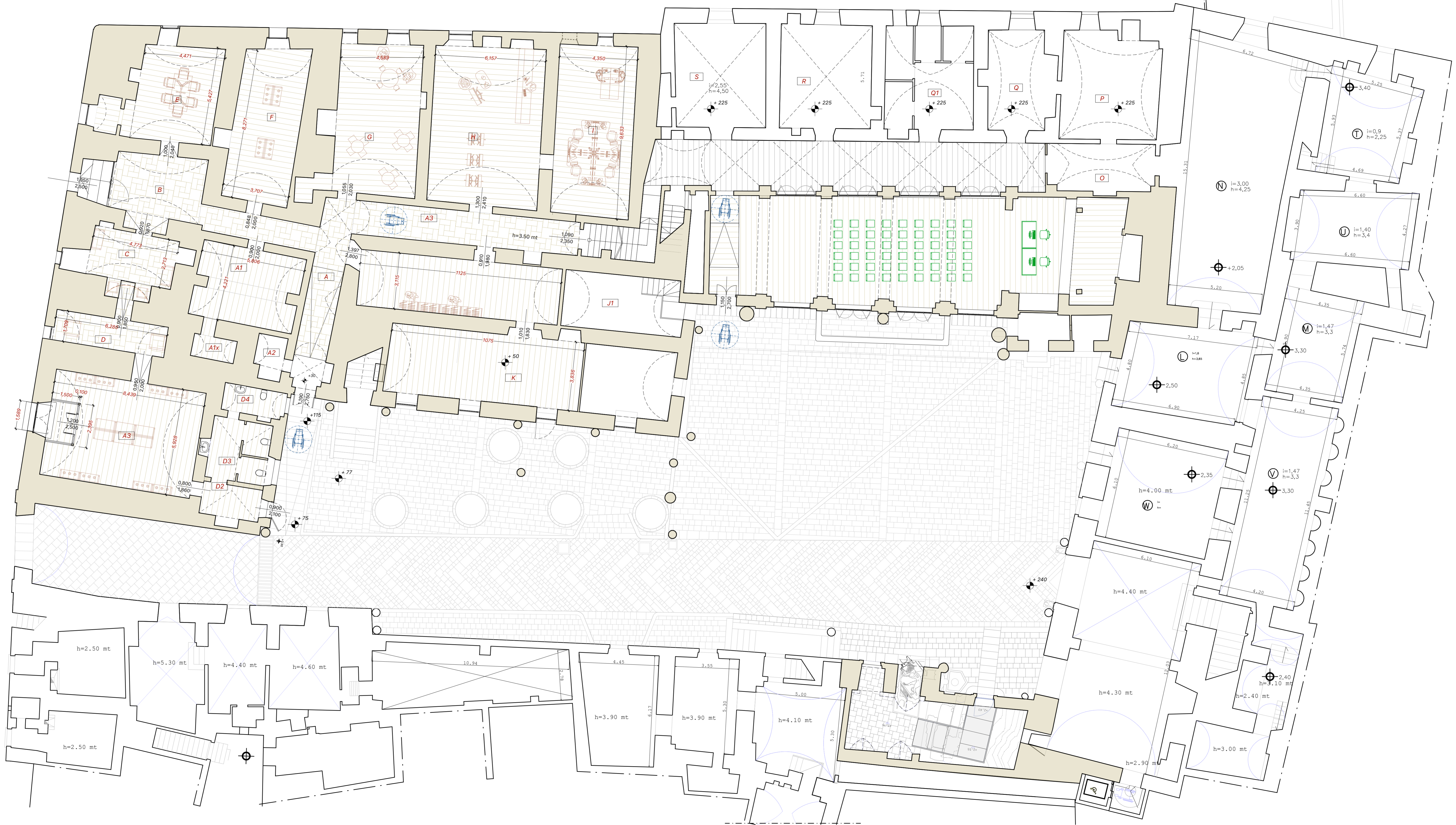
LAYOUT PIANTA PIANO TERRA scala 1:100
